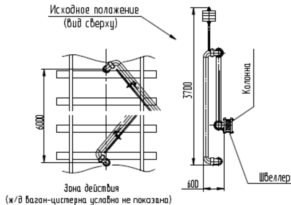
Монтажная схема
