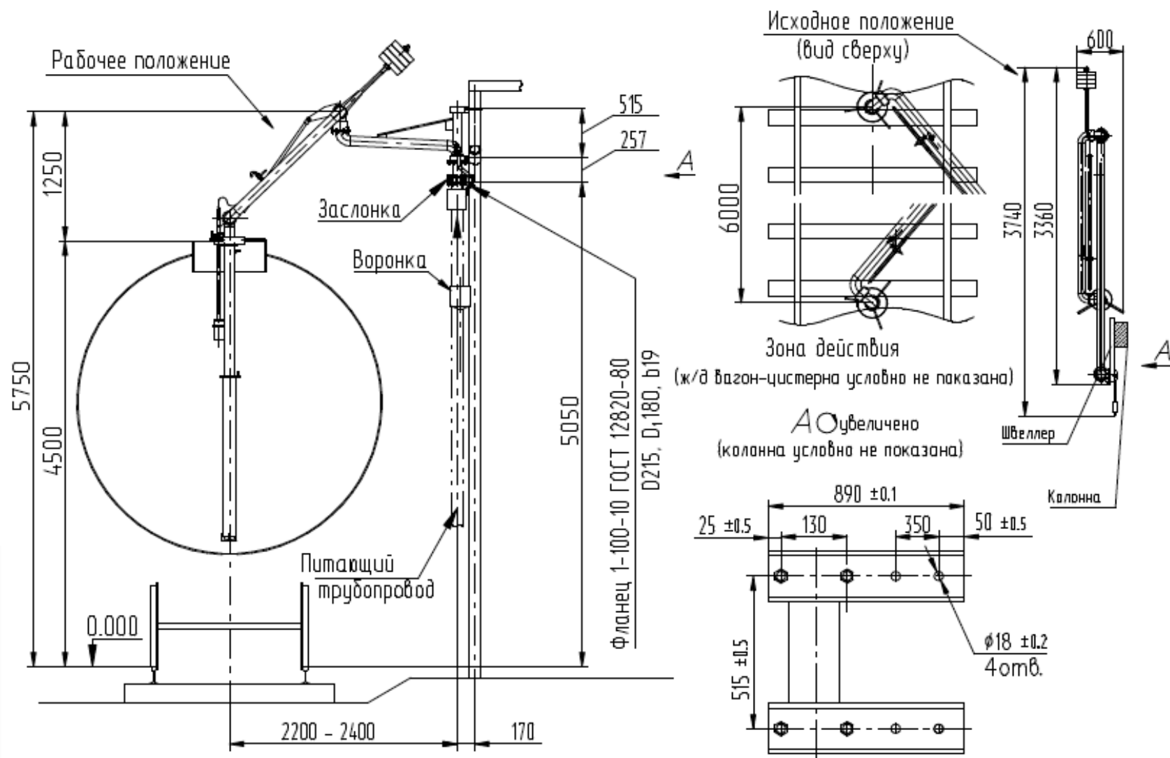
Монтажная схема
