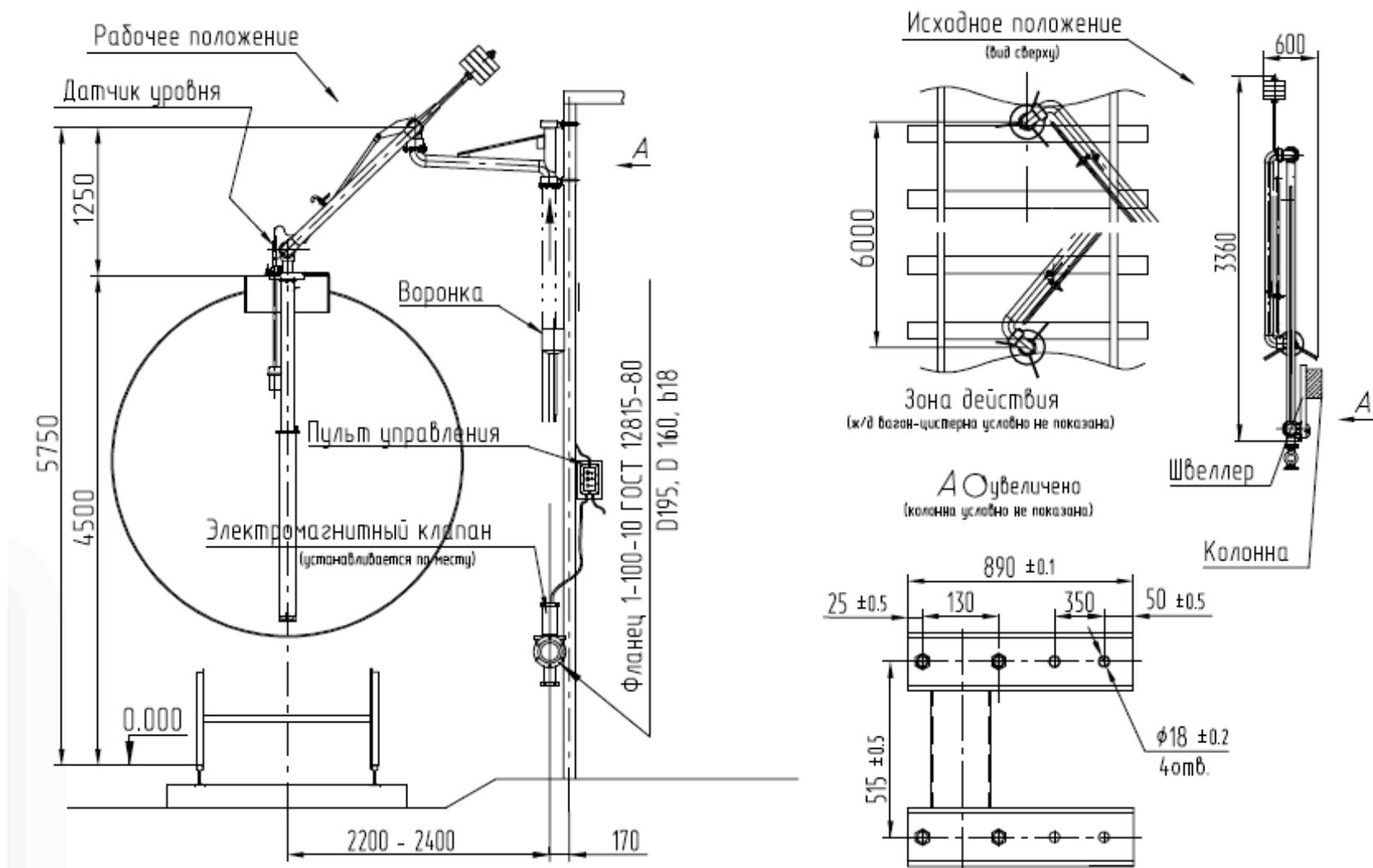
Монтажная схема
